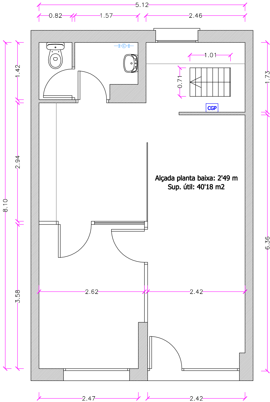
Planta Baixa L63 (Avinguda Burgos 16)
