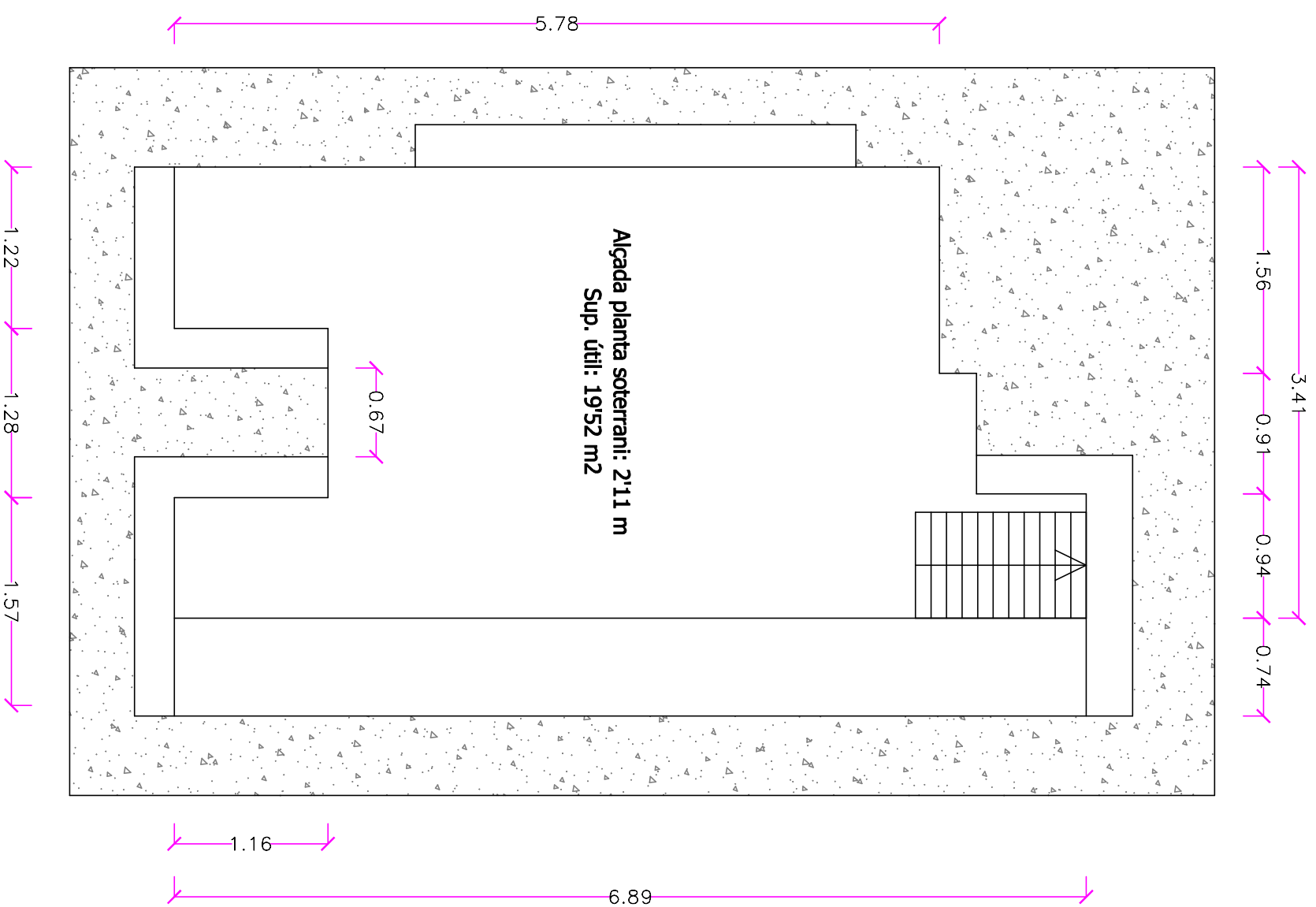
Planta Soterrani L15 (Carrer Porto 7)
