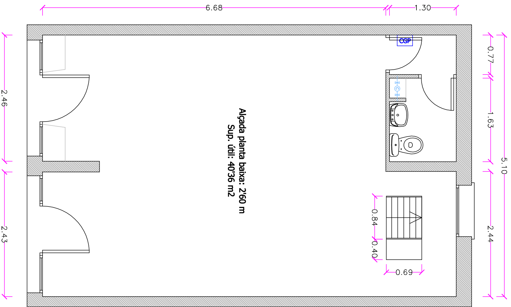
Planta Baixa L15 (Carrer Porto 7)
