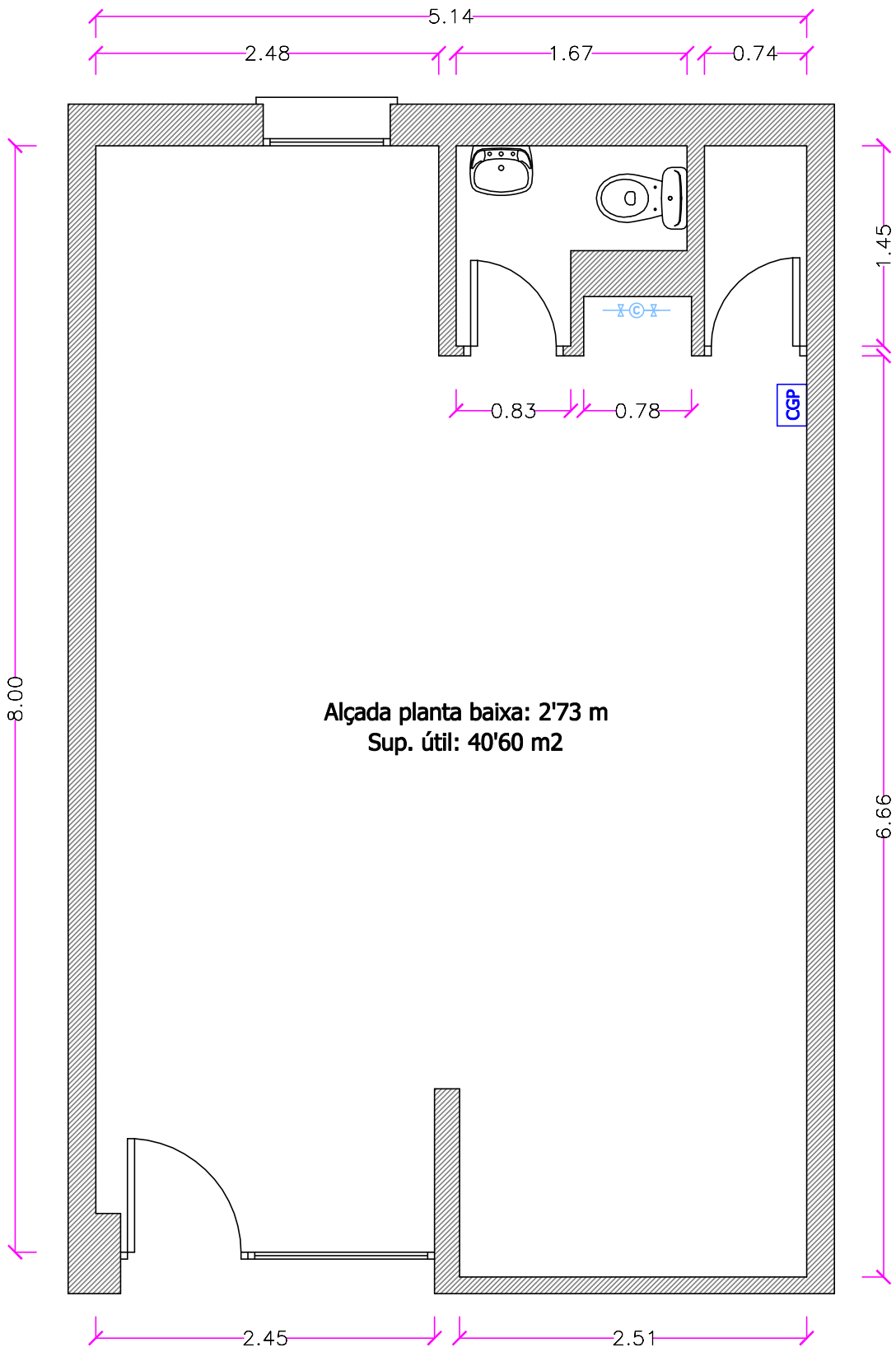
Planta Baixa L112 (Avinguda Eivissa 6)
